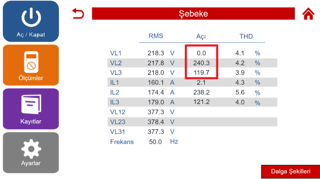
Şekil 46: Şebeke açılarının kontrolü
