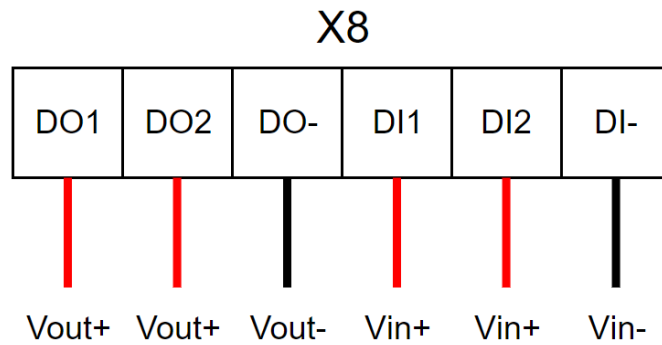
Şekil 11: X8 klemensinin haritalandırılması
