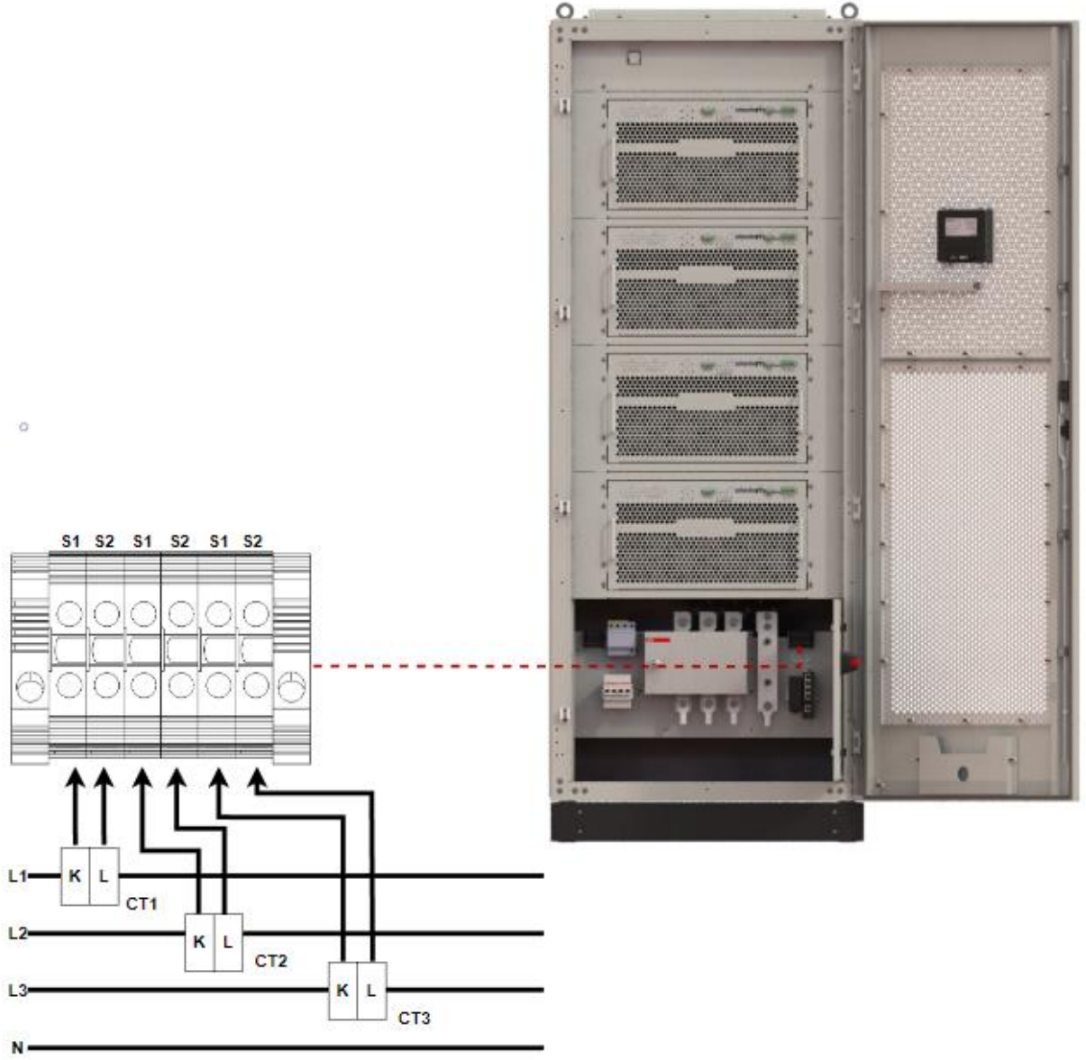
Şekil 9: AHF pano tipi akım trafosu bağlantısı
