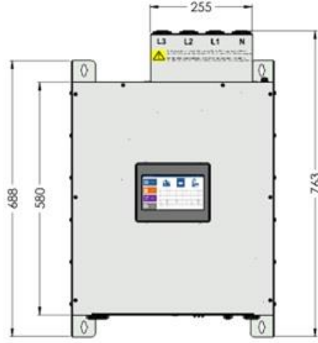
Şekil 1: AHF duvar tipi ölçüleri
