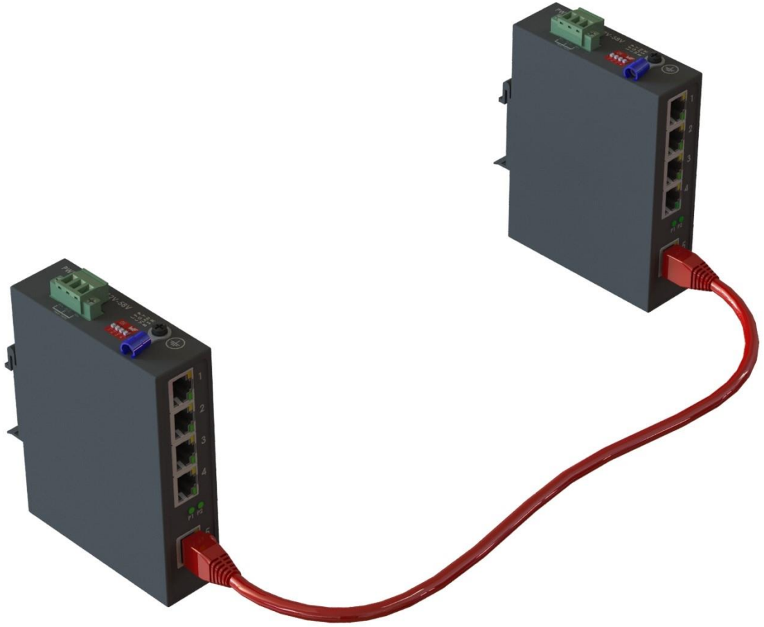
Şekil 17: İki ayrı panolarda bulunan switch ortaklama işlemi
