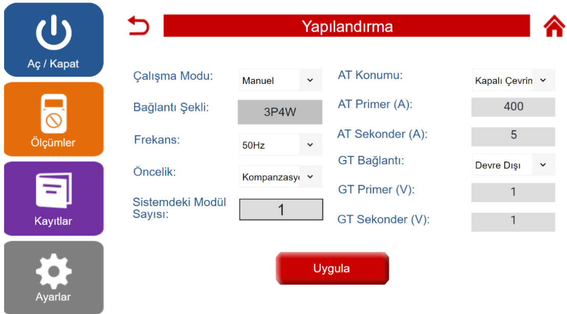
Şekil 25: “Yapılandırma” menüsü
