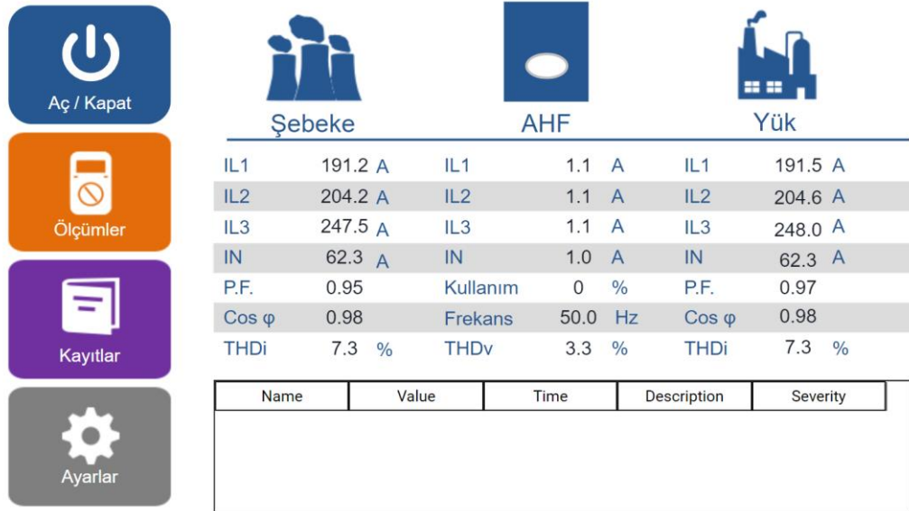
Şekil 18: “Ana Ekran”
