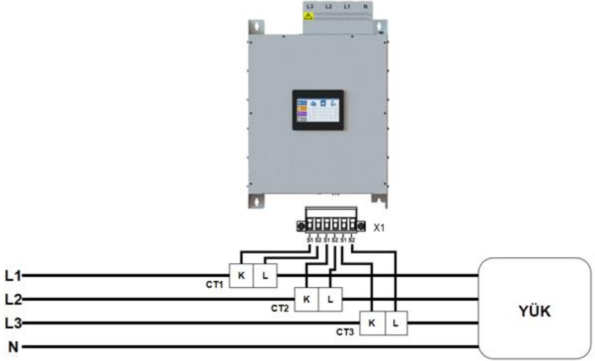
Şekil 8:AHF Duvar Tipi Akım trafosu bağlantısı
